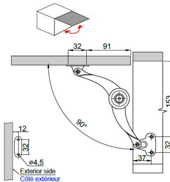
Lift-off door / Ouverture de porte 90°
